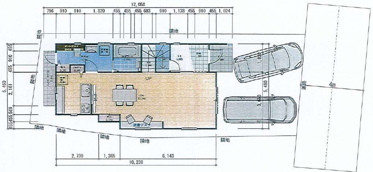
1階 縮尺 1/100
