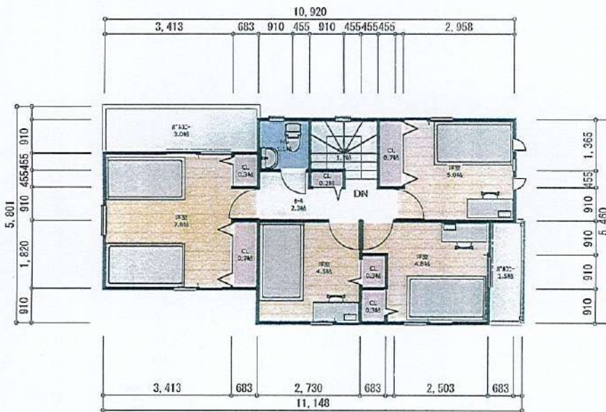
2階 縮尺 1/100
